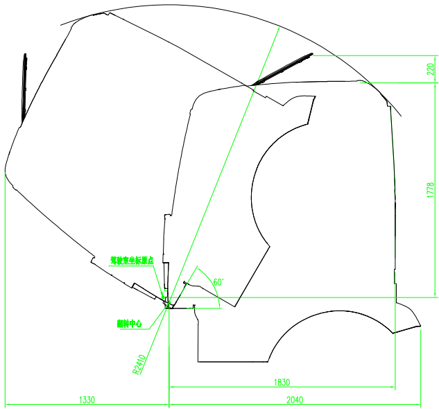
TX-M 驾驶室侧视图 1:10
